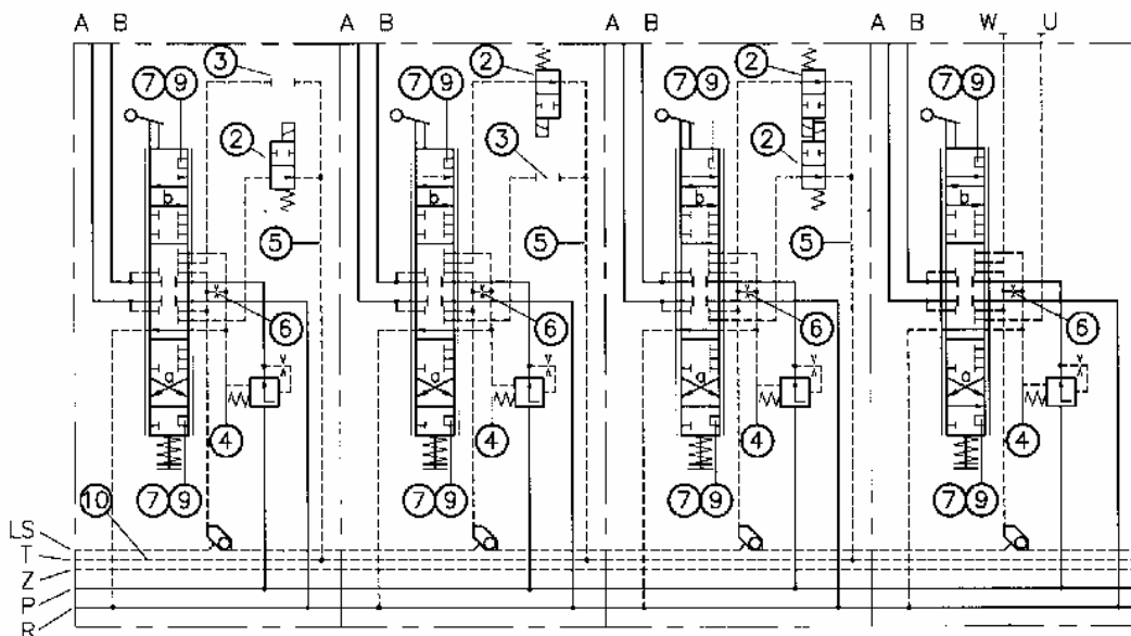
F1:型总装原理图
