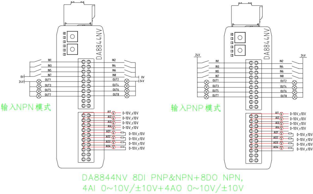
JKPN-DA8844NV 模块接线图：
