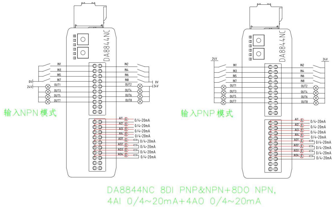
JKPN-DA8844NC 模块接线图：
