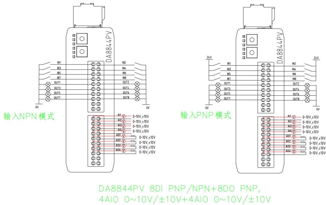
JKPN-DA8844PV 模块接线图：
