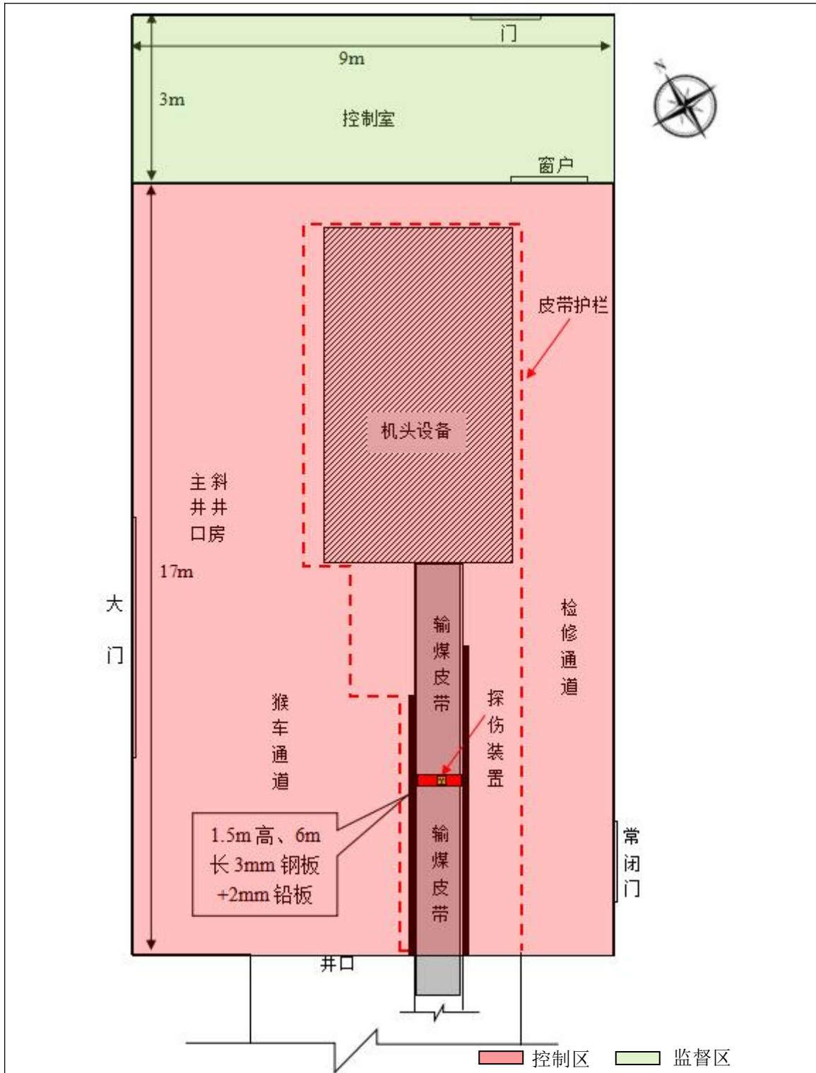
图 5.1 辐射防护分区示意图
