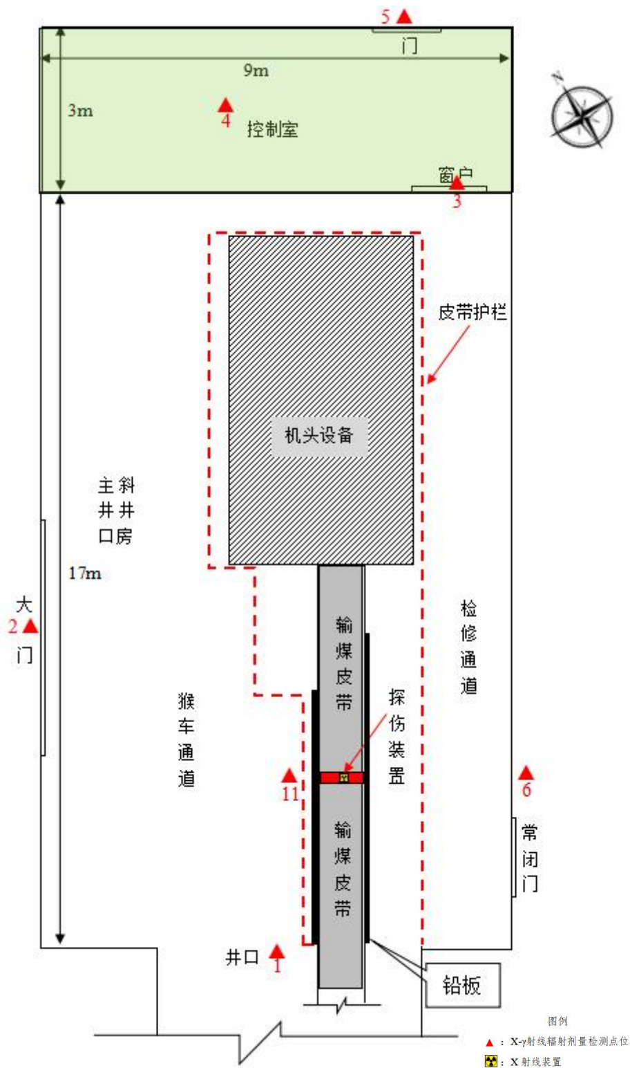
图 7.1 监测点位示意图 1
