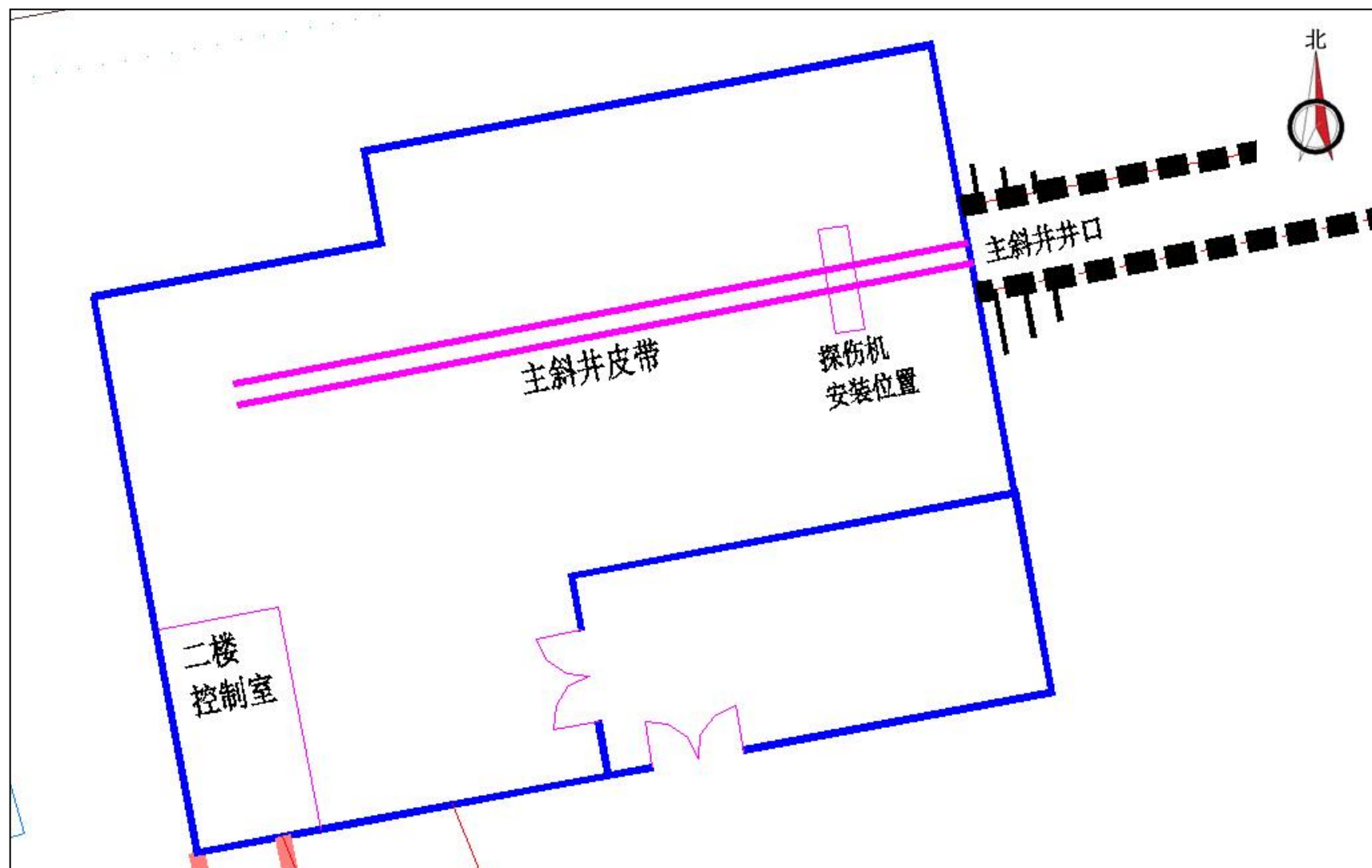
主斜井井口房平面布置示意图
