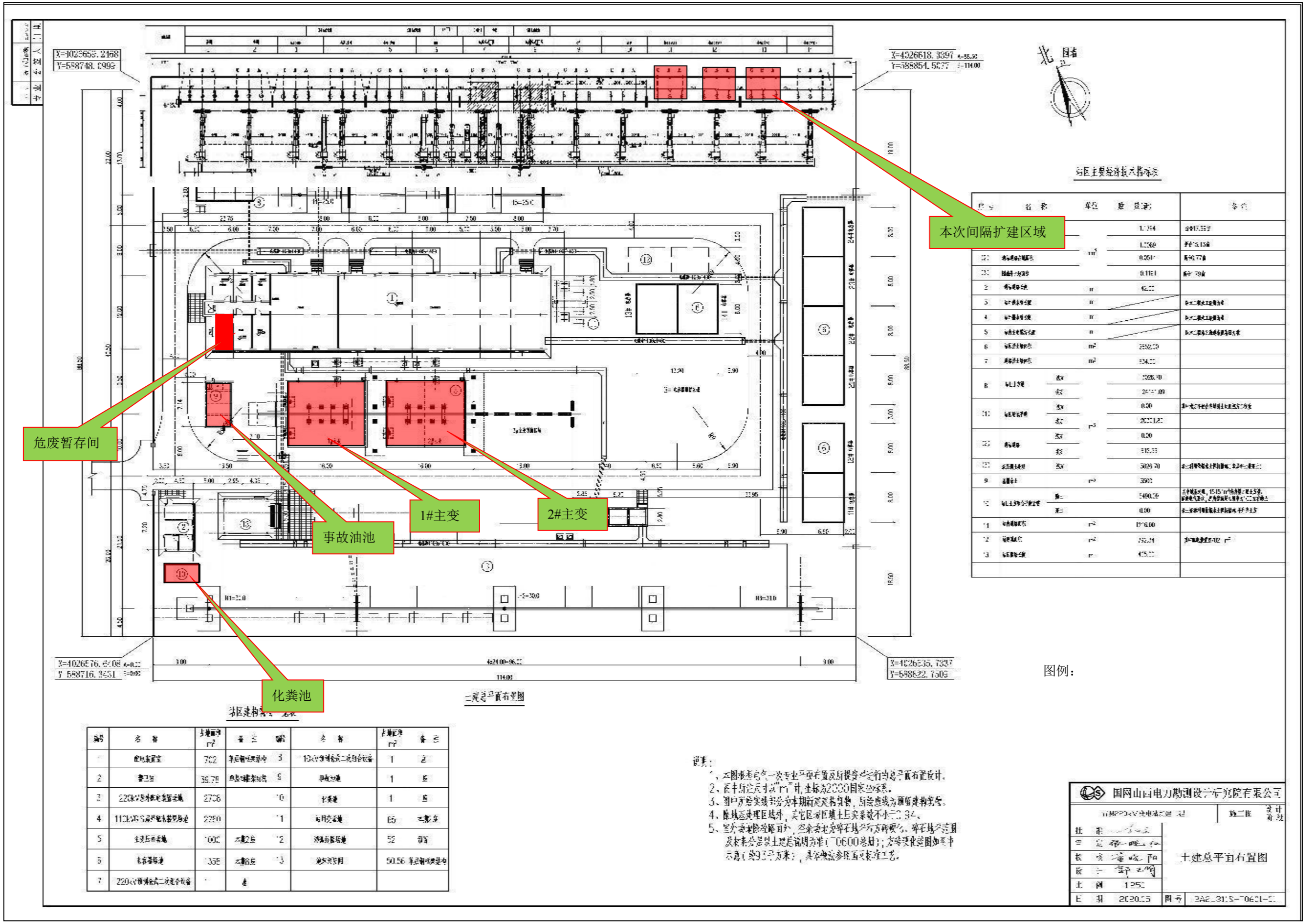
附图3 相如220kV变电站平面布置示意图
