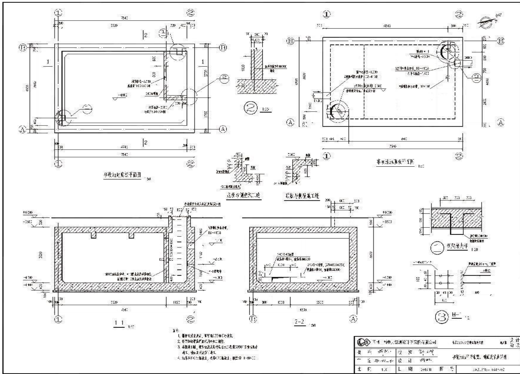
附图5 事故油池平剖图
