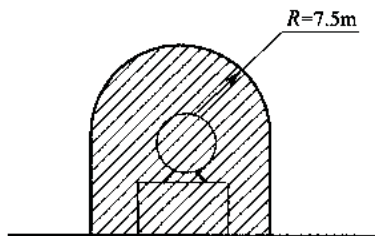
图 C.0.13 露天(棚)设置的 CNG 压缩机、阀门、法兰或类似附件的爆炸危险区域划分
